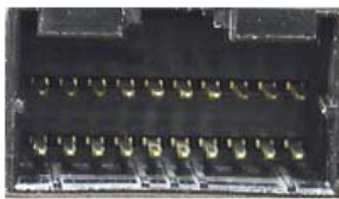
Разъем Subaru тип 10+10
