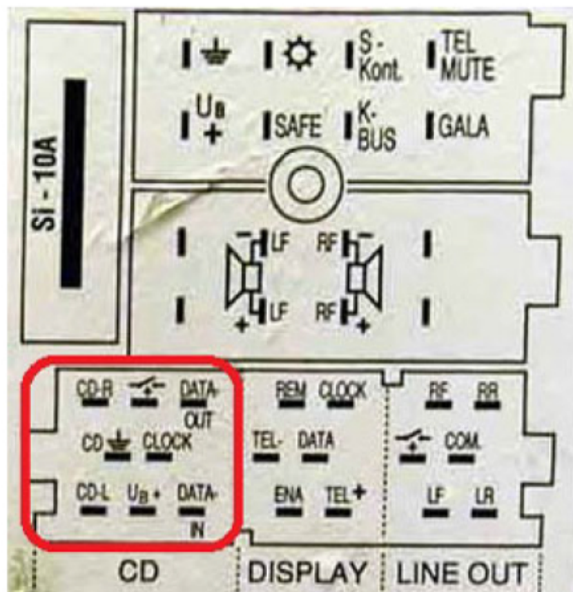
Разъем Volkswagen тип 8-pin (VAG, Mini-ISO)
