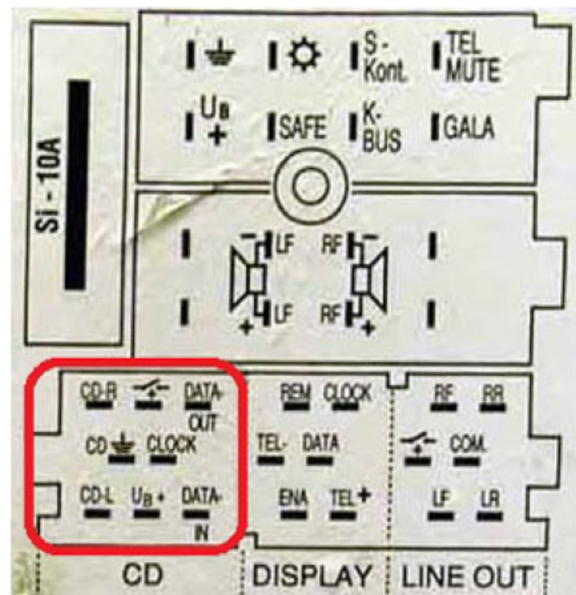
Разъем Skoda тип 8-pin (VAG, Mini-ISO)
